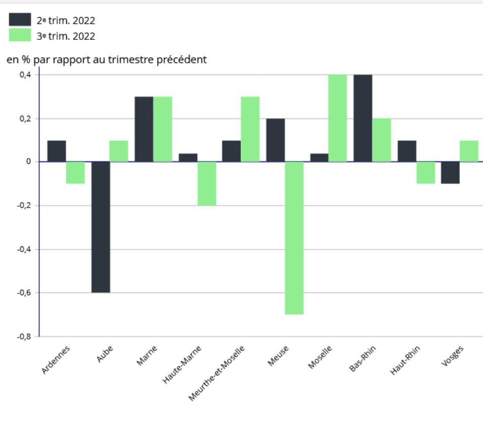
Figure 4 – Évolution de l'emploi salarié total par département
